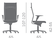
Schienale alto - High back
