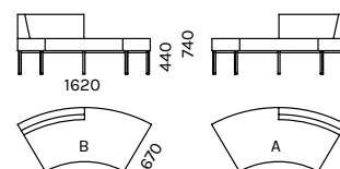
ZK-DKA-MJ, ZK-DKB-MJ
