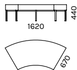
ZK-PK90-MJ
