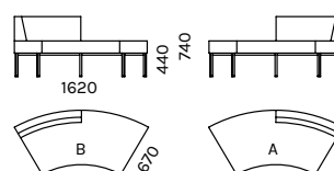
ZK-DKA-MJ, ZK-DKB-MJ
