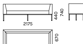
ZK-D3AB-MJ
