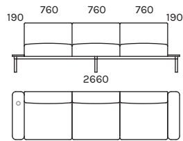
N28 LAR321-LALP2-LAIS2-LAIS2-LAIS2-LALP1
